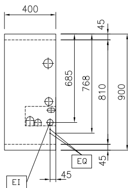
Boven aanzicht
